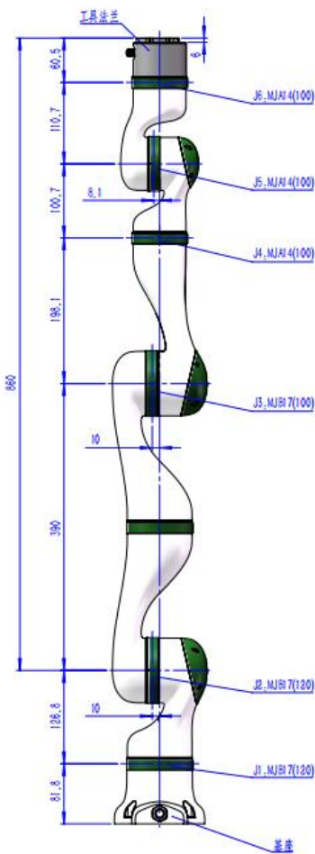
TC6-R3 尺寸
