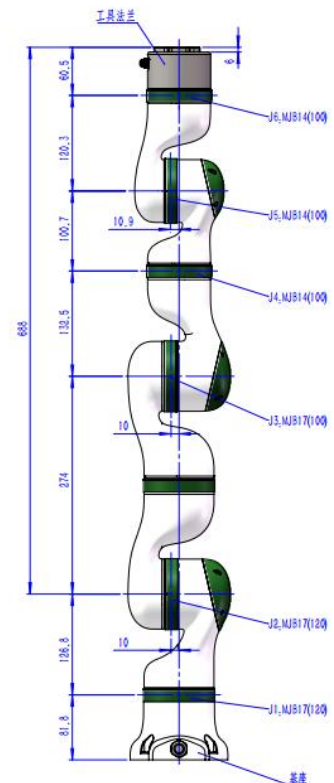
TC6-R3S 尺寸
