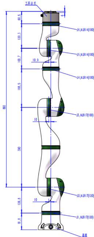
TC6-R3B 尺寸
