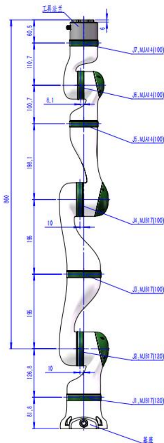
TC7-R3 尺寸
