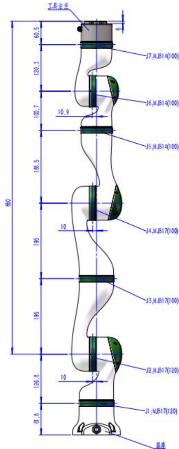
TC7-R3B 尺寸
