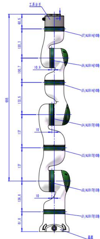
TC7-R3S 尺寸
