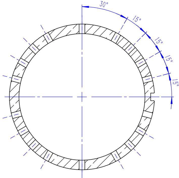
安装孔位分布图 Installation Hole Distribution Diagram
