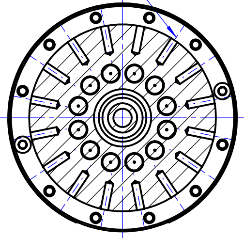
剖面 A-A
