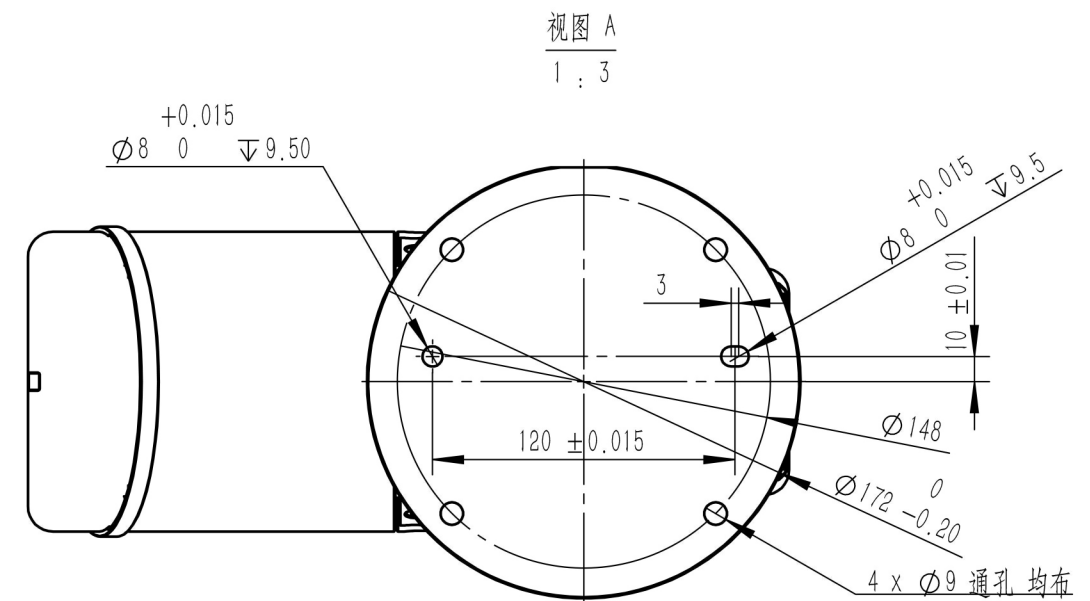
底座安装孔位示意图
