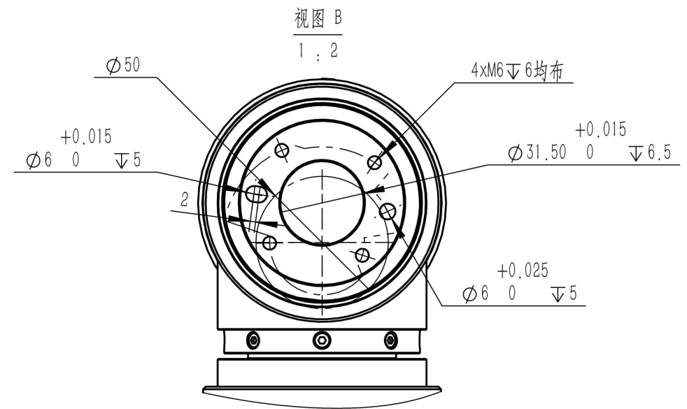
末端输出法兰安装孔位示意图
