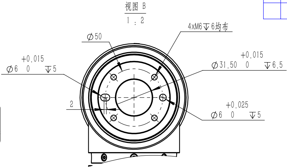
末端输出法兰安装孔示意图
